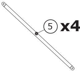
Ø6x440mm
